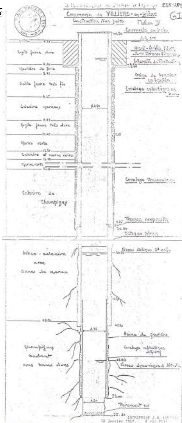
Figure 5-1: Coupe technique du P1 de Villiers-en-Bière
