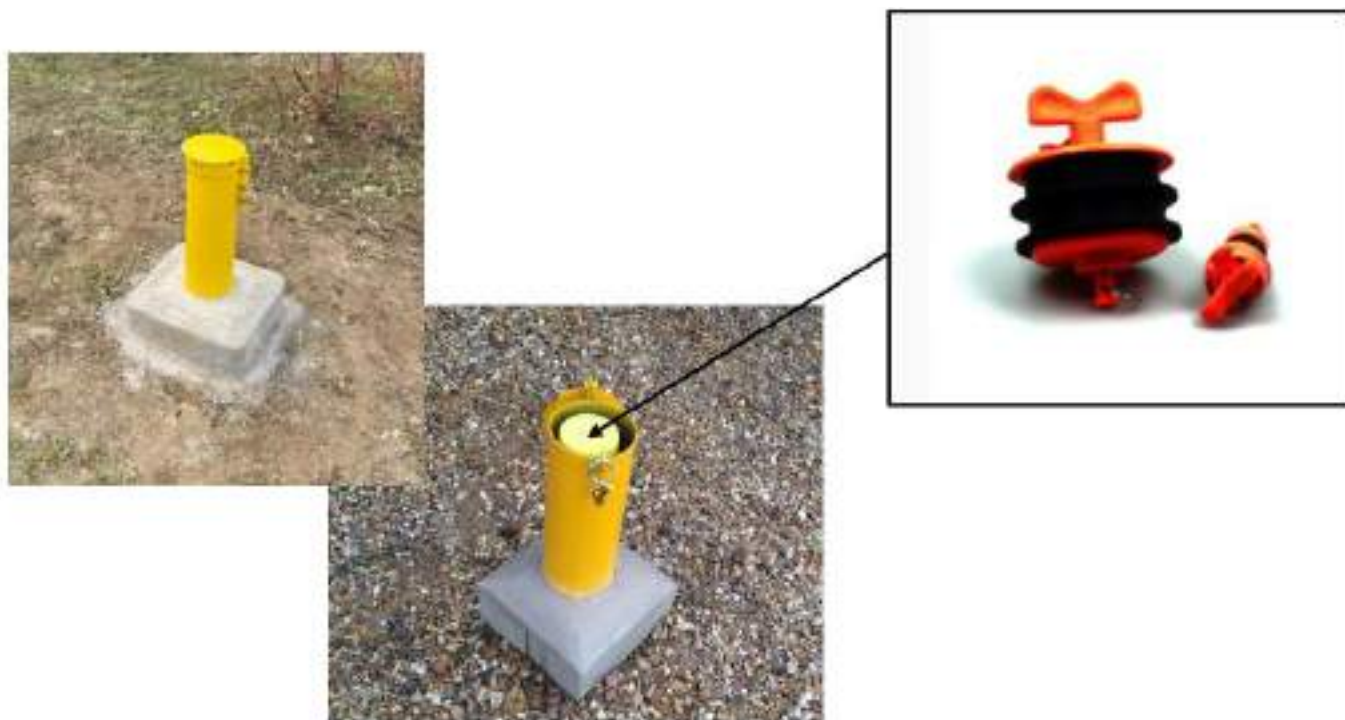
Figure 13 – Exemple de la partie hors sol d'un piézomètre (aménagement avec fermeture sécurisée par capot acier pris dans la dalle périphérique à pentes divergentes) et bouchon étanche pour obturation du tube PVC
