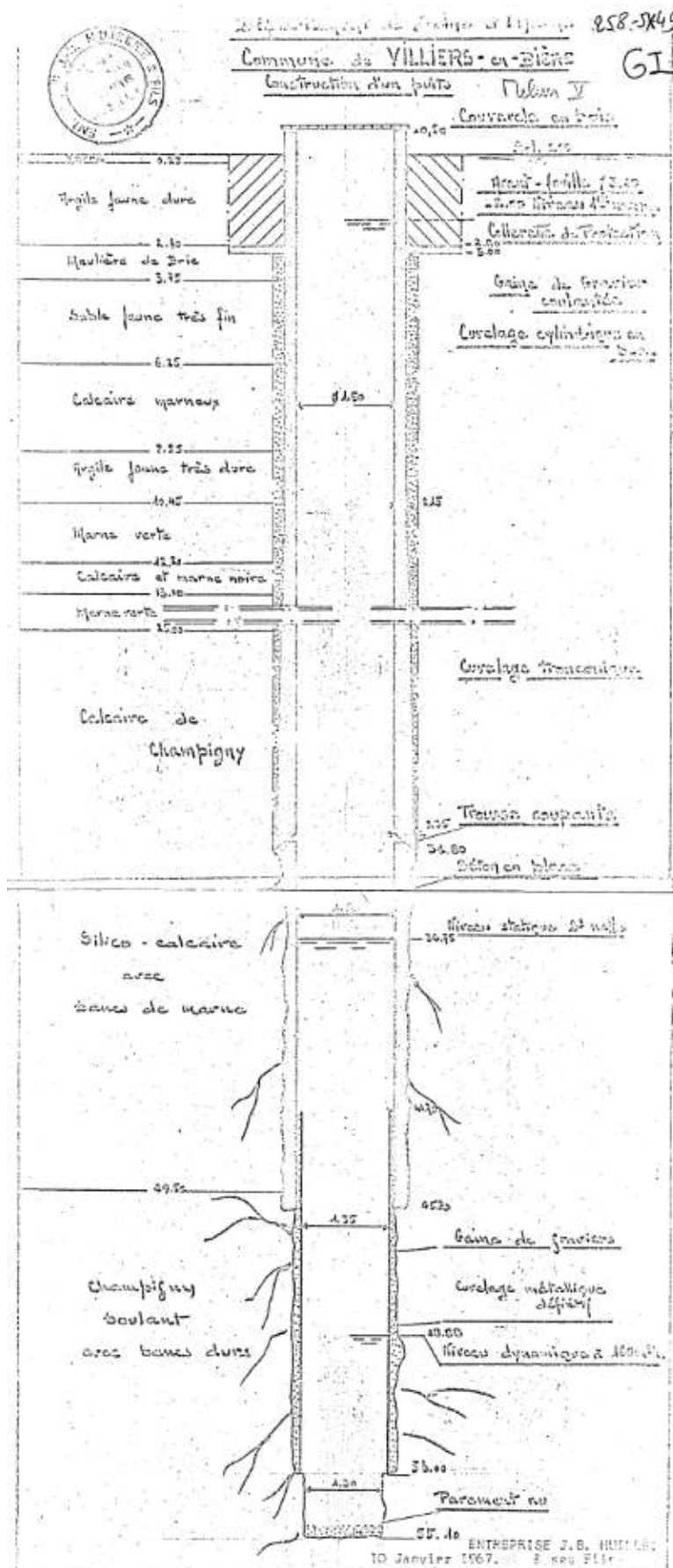
Figure 3 - Coupe technique et géologique de référence du Forage Villiers 1
