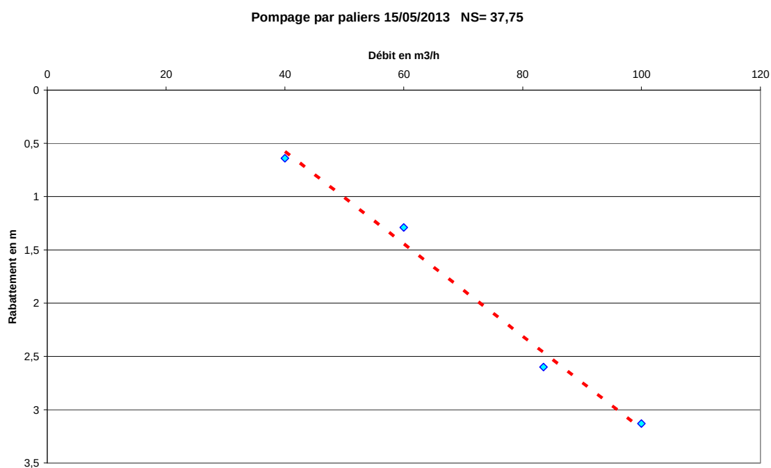
Figure 5-2: Résultats de l'essai de pompage par paliers
