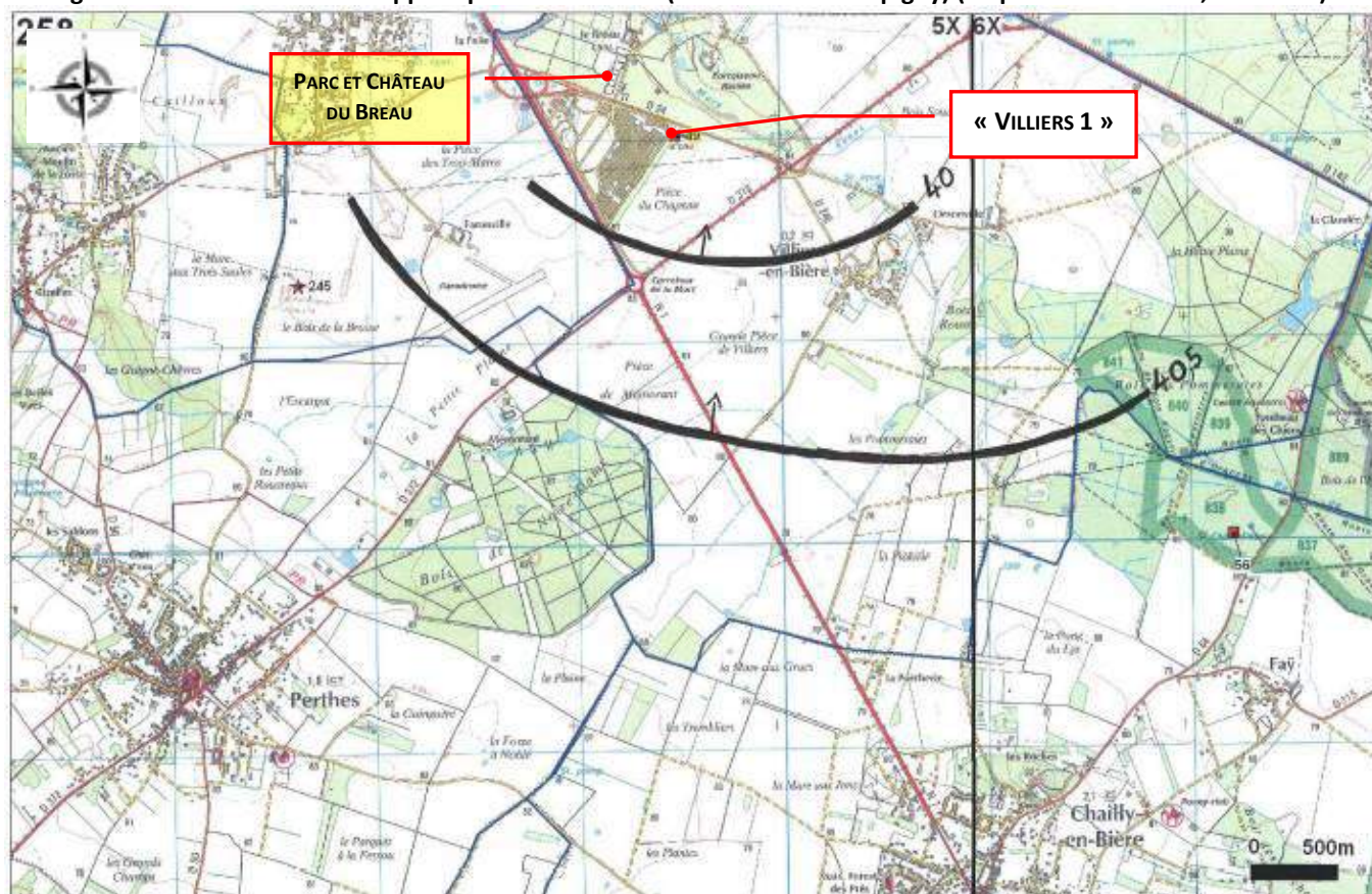
Figure 6 - Piézométrie de la nappe captive de l'Eocène (Calcaires de Champigny) (d'après Archambault, Mai 2013)
