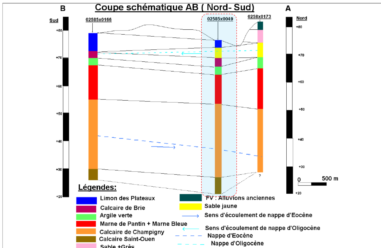
Figure 5 – Coupe corrélatrice Nord-Sud (Source Archambault Conseil, Rapport 2013)
