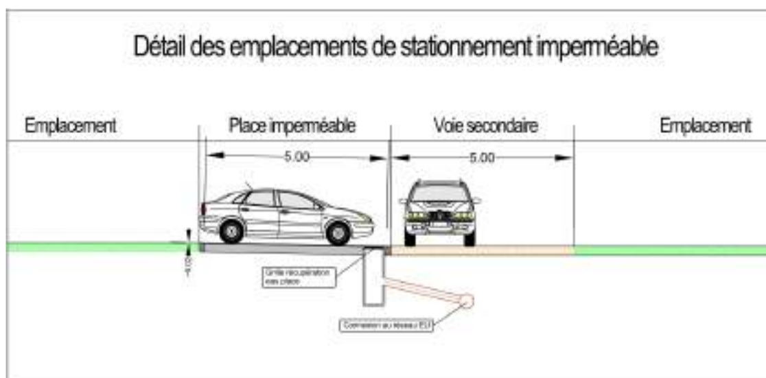
Figure 9 – Aménagements particuliers des sites de stationnement des véhicules du quotidien
