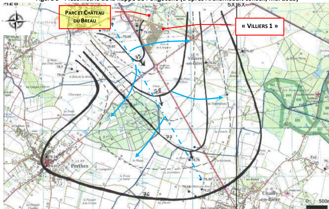
Figure 5 - Piézométrie de la nappe de l'Oligocène (d'après Archambault conseil, Mai 2013)
