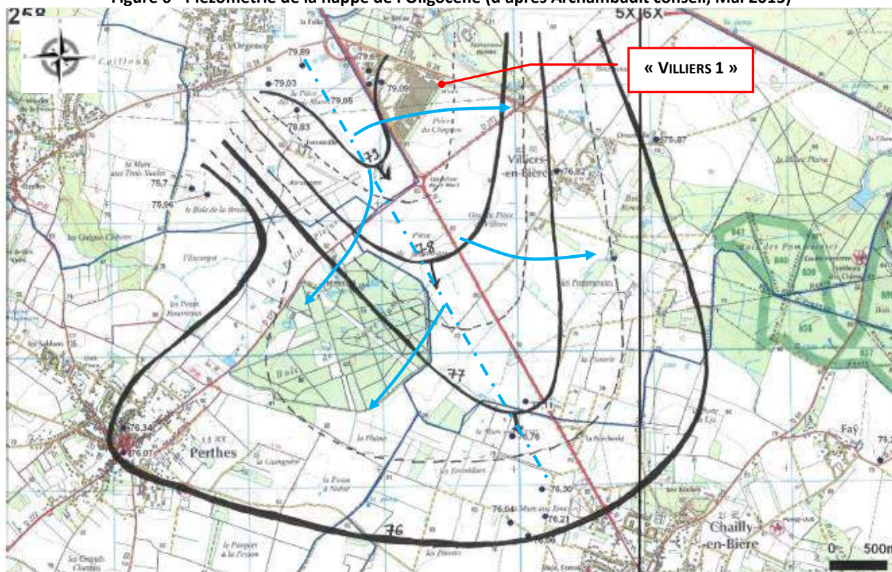
Figure 6 - Piézométrie de la nappe de l'Oligocène (d'après Archambault conseil, Mai 2013)
