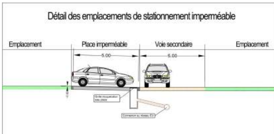
Figure 08 : détail des emplacements de stationnement imperméable et du système de collecte des eaux
