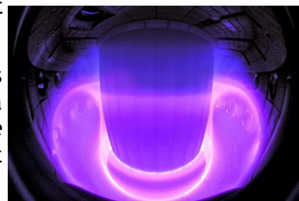
Photo du tokamak, réalisée par l'Ecole Polytechnique Fédérale de Lausanne (EPFL). Crédits Curdin Wüthrich/SPC/EPFL
